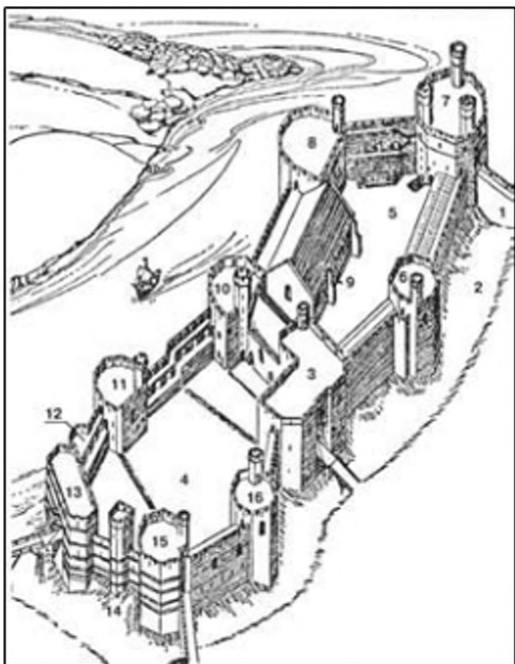
Королівський замок в Англії: 1 – міський жур, 2 – захисний рів, 3 – королівські ворота, 4 – зовнішній двір замку, 5 – внутрішній двір замку, 6 – колодезна вежа, 7 – орхіна вежа, 8 – вежа королеви, 9 – основний зал, 10 – вежа управителя, 11 – Чорна вежа, 12 – вежа-водосховище, 13 – ворота королеви, 14 – сторожова вежа, 15 – північно-східна вежа, 16 – колірна вежа
