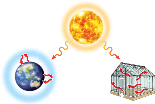
Мал. 34. Схематичне зображення парникового ефекту
