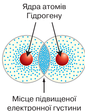
Мал. 58. Прекривання s -орбіталей з утворенням спільної електронної пари в молекулі водню
