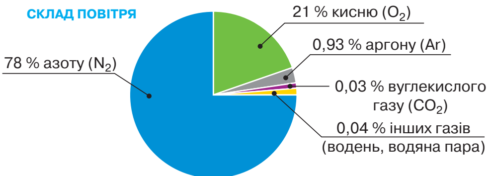
Мал. 12. Об'ємний склад повітря
