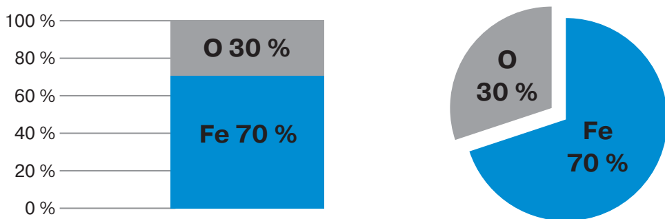
Мал. 4. Масові частки елементів у ферум(III) оксиді \text{Fe}_2\text{O}_3
