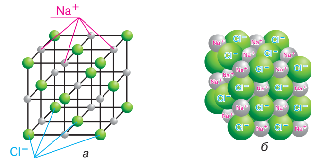
Мал. 64. Кристалічні ґратки (а) і модель йонного кристала (б) натрій хлориду
