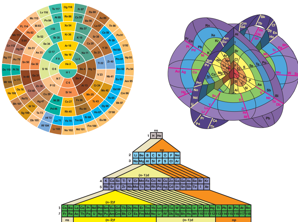
Мал. 51. Деякі форми періодичної таблиці
