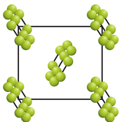
Кристалічні ґратки нафталіну
