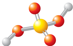
Мал. 5. Модель молекули сульфатної кислоти
