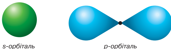
Мал. 42. Схематичне зображення s- і p-орбіталей атома
