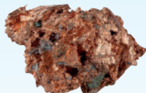
Мідна руда
