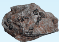
Залізна руда
