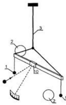
Рис. 2.16. Досліди Кавендіша
