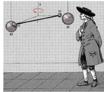
Рис. 2.16. Досліди Кавендіша
