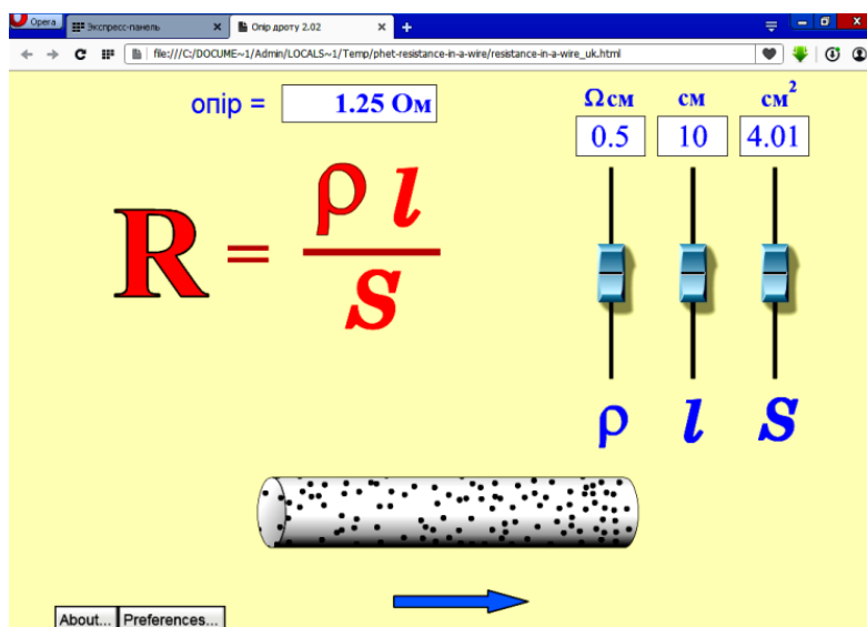
Рис. 2.11. Модель для розв'язування задач із теми «Питомий опір провідника»
