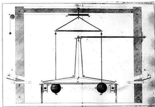
Рис. 2.15. Крутильні терези
