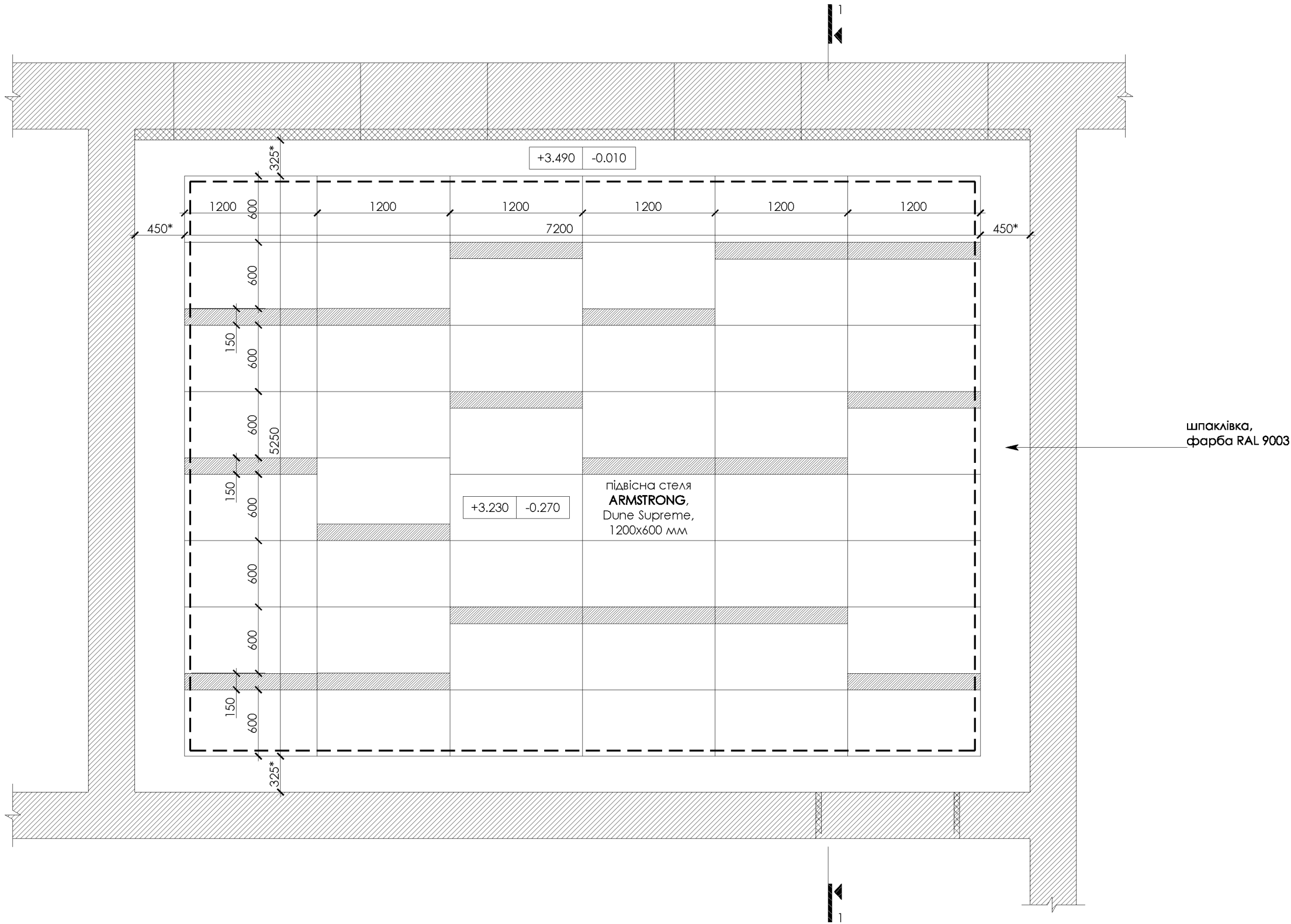
План стелі з розміщенням літарів, М 1:40
