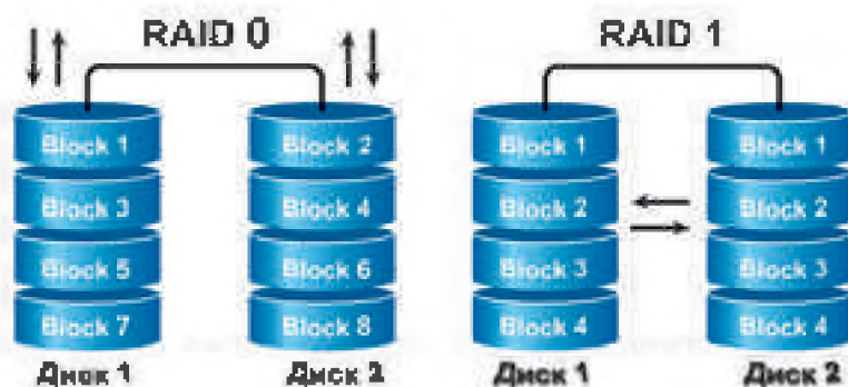
Fig. 4.15. Schema funcționării RAID-masivelor de nivelul 0 și nivelul 1
